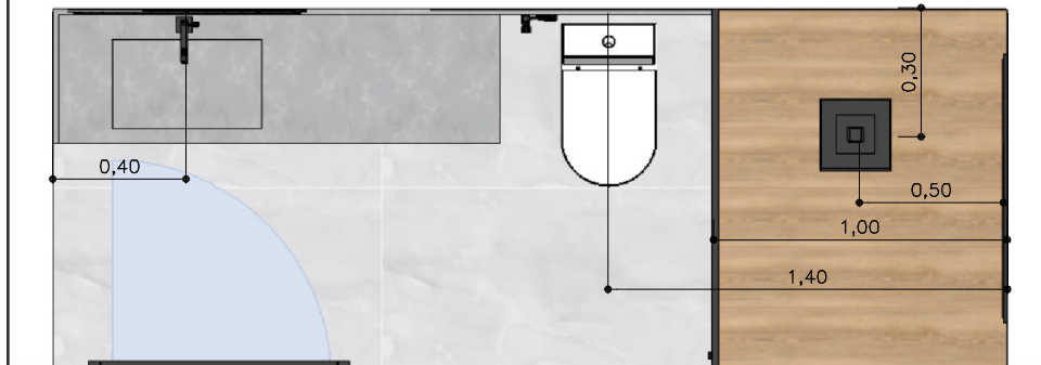
PONTOS HIDRÁULICOS - SUÍTE INFANTIL
