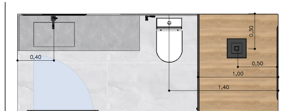
COTAS PRINCIPAIS - BANHO SUÍTE INFANTIL
