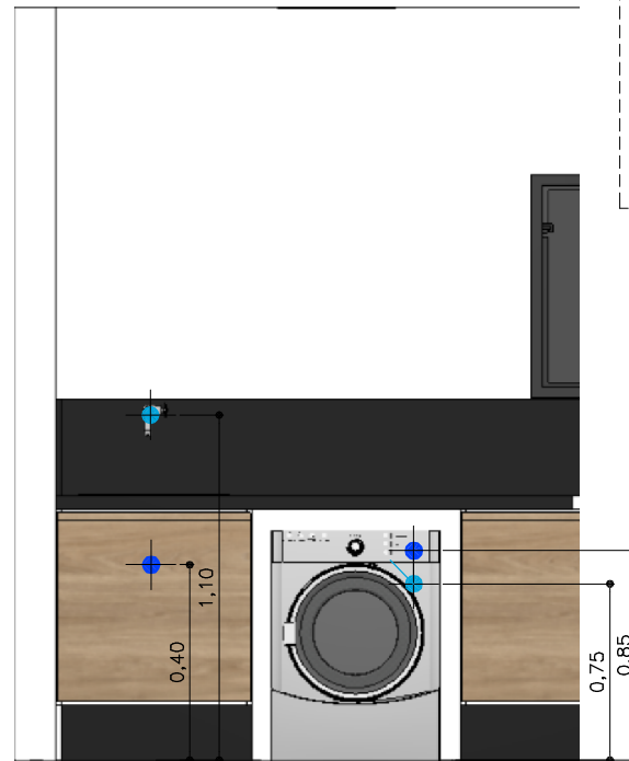
PONTOS HIDRÁULICOS - ÁREA DE SERVIÇO
