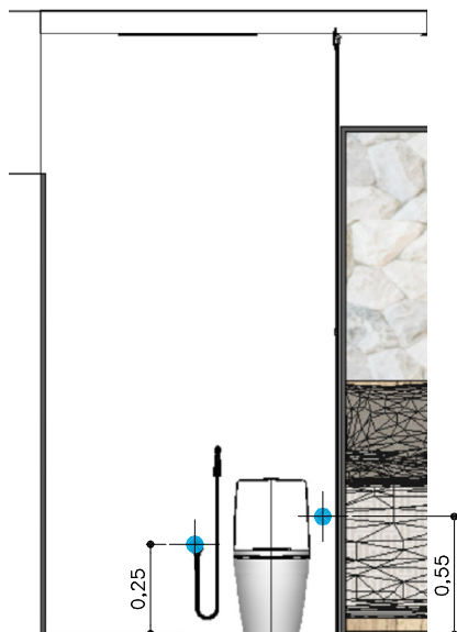
PONTOS HIDRÁULICOS - SUÍTE CASAL
