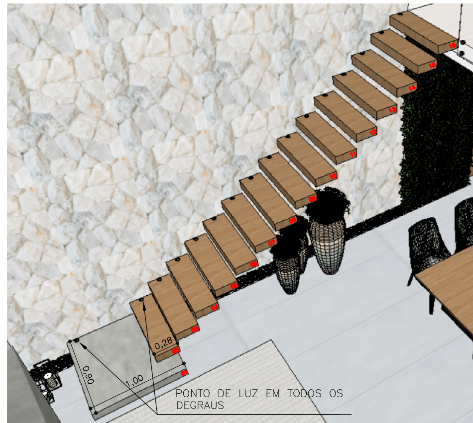
DETALHE ESCADA
