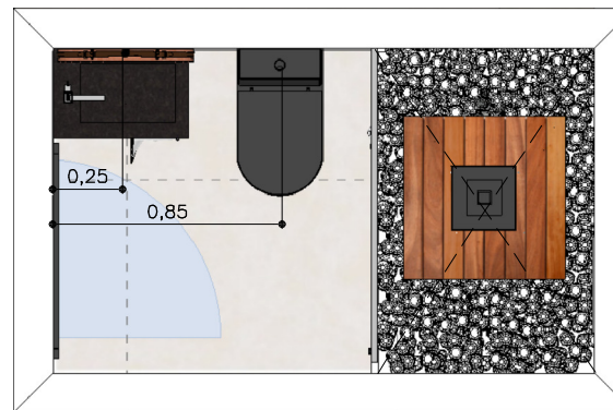
PONTOS HIDRÁULICOS - BANHO GOURMET
