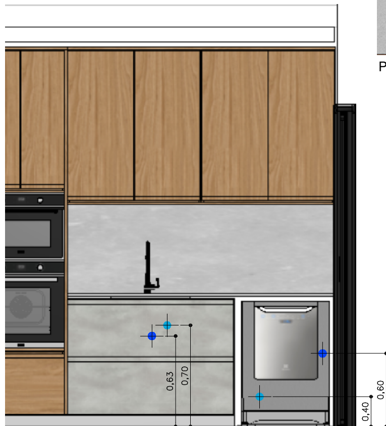
PONTOS HIDRÁULICOS - COZINHA
