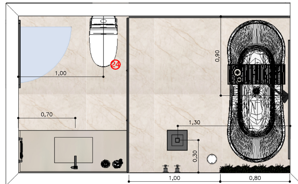
COTAS PRINCIPAIS - BANHO SUÍTE CASAL
