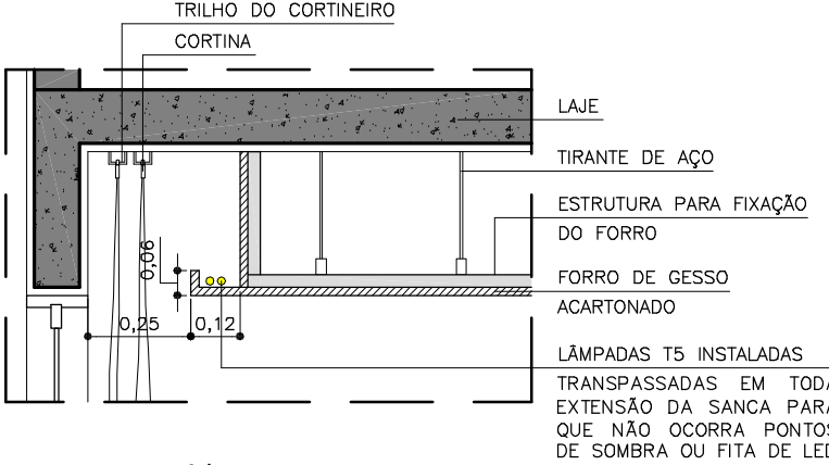
DETALHE 02 - CORTINEIRO ILUMINADO ESCALA 1:20
