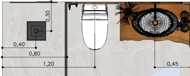
PONTOS HIDRÁULICOS - BANHO TÉRREO
