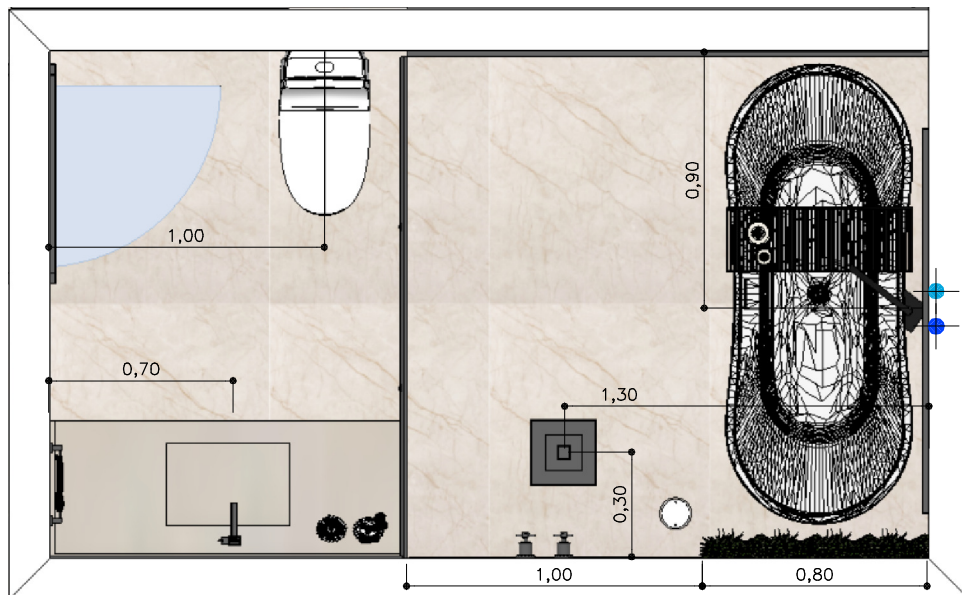
PONTOS HIDRÁULICOS - SUÍTE CASAL
