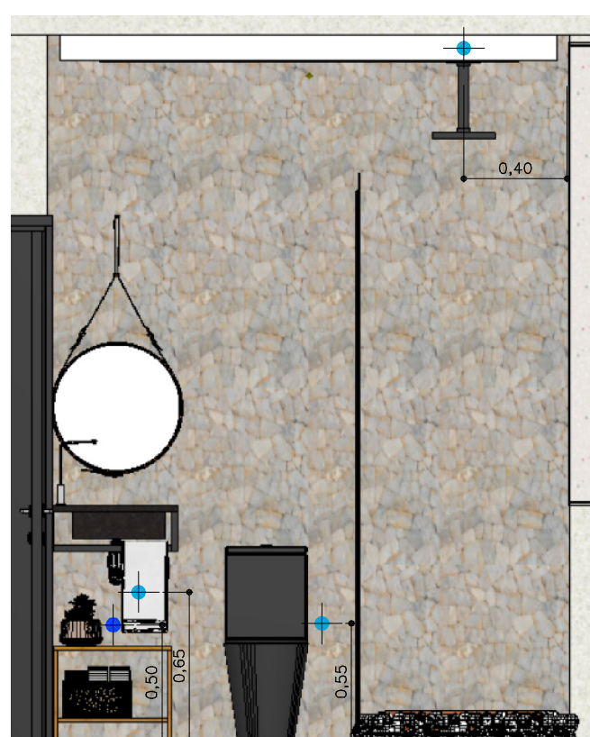
PONTOS HIDRÁULICOS - BANHO GOURMET
