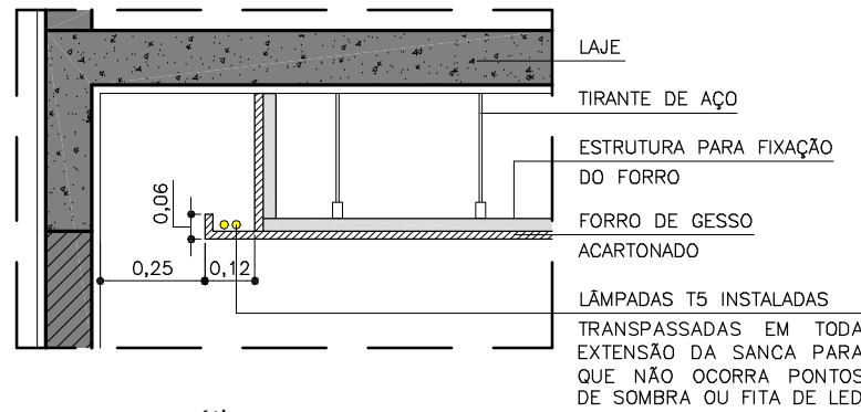
DETALHE 01 - RASGO ILUMINADO ESCALA 1:20
