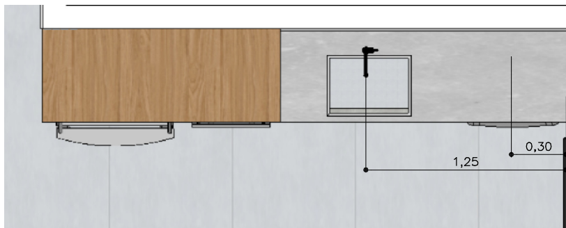
PONTOS HIDRÁULICOS - COZINHA
